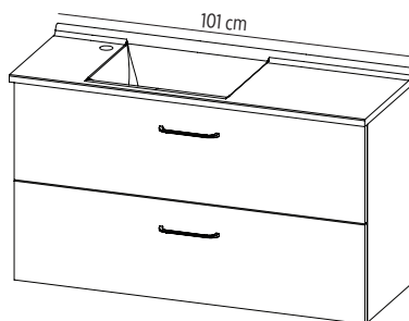
MEUBLE 2 TIROIRS VASQUE À GAUCHE L 100 cm
